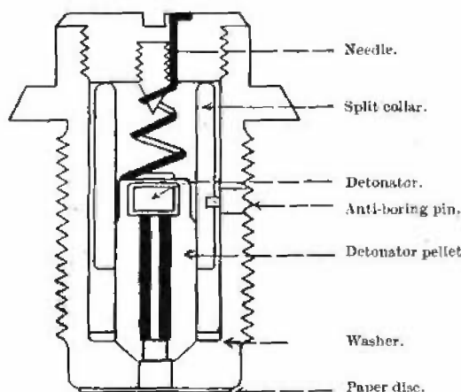
Fig. 78. FUZE, PERCUSSION, Q.F., 1-PR. Scale = \frac{1}{2} .
