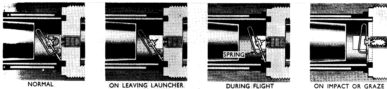
Fig. 26 Action of Striker
