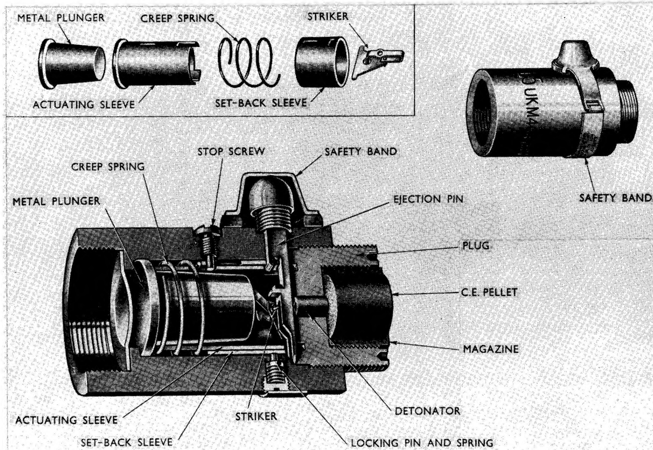
Fig. 16 FUZE, L5. U.K. M404 Mark I
