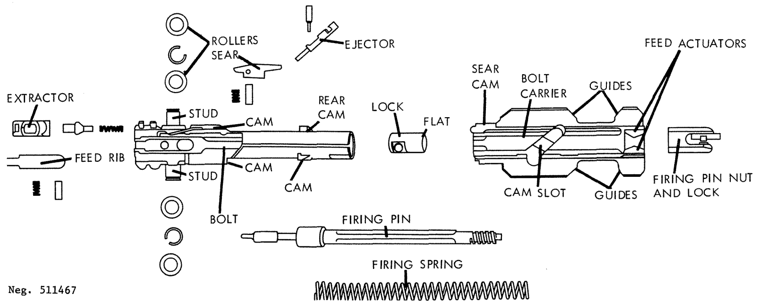
Figure 168. MG34 bolt.
