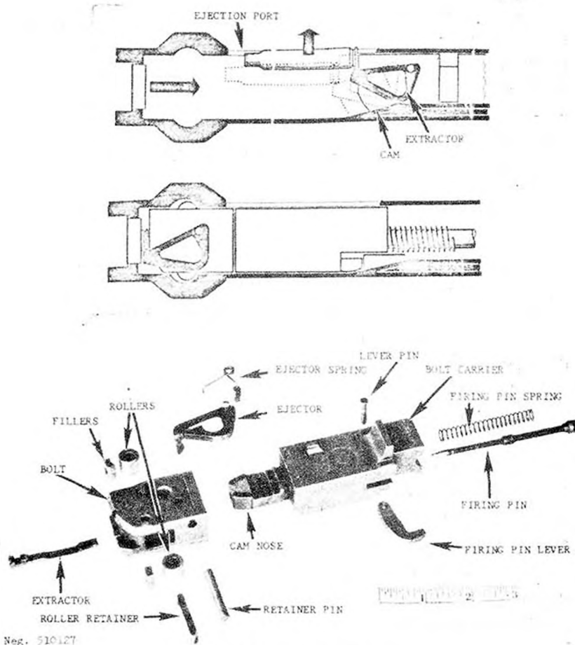
Figure 128. StG 57 bolt.
