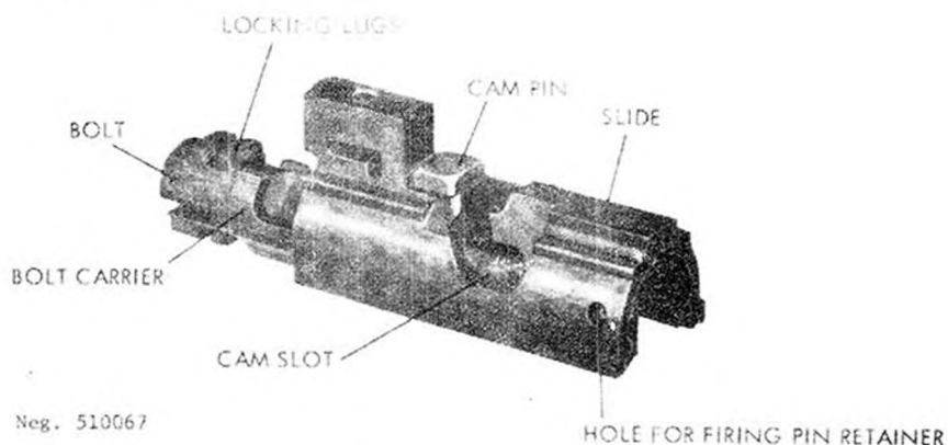
Figure 68. C.A.L. bolt.
