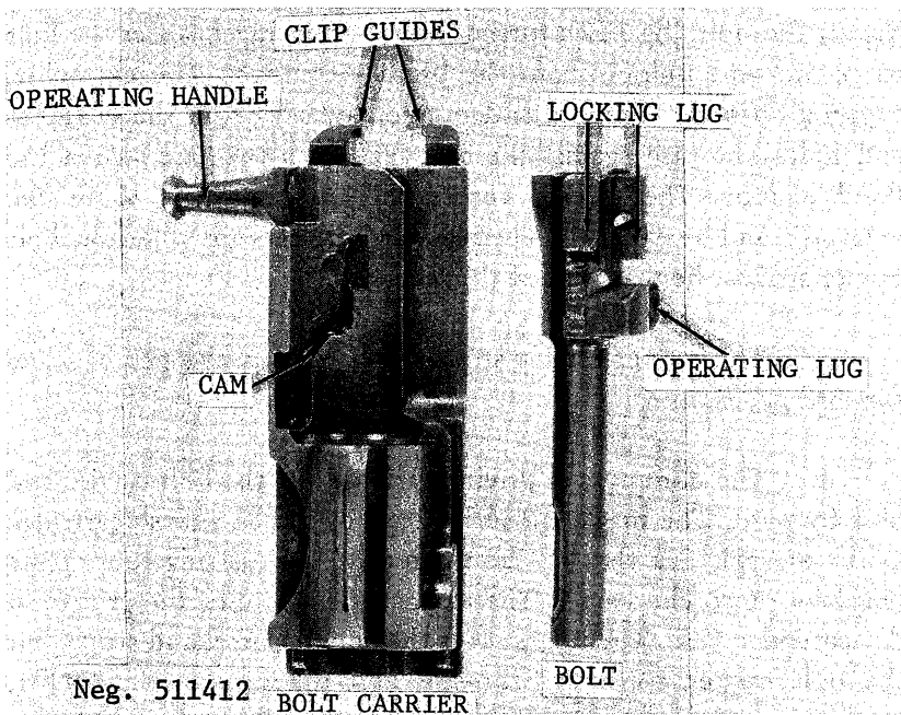
Figure 112. Type 68 bolt.
